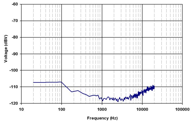
NOISE FFT
