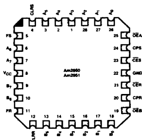
Chip-Pak™ L-28
