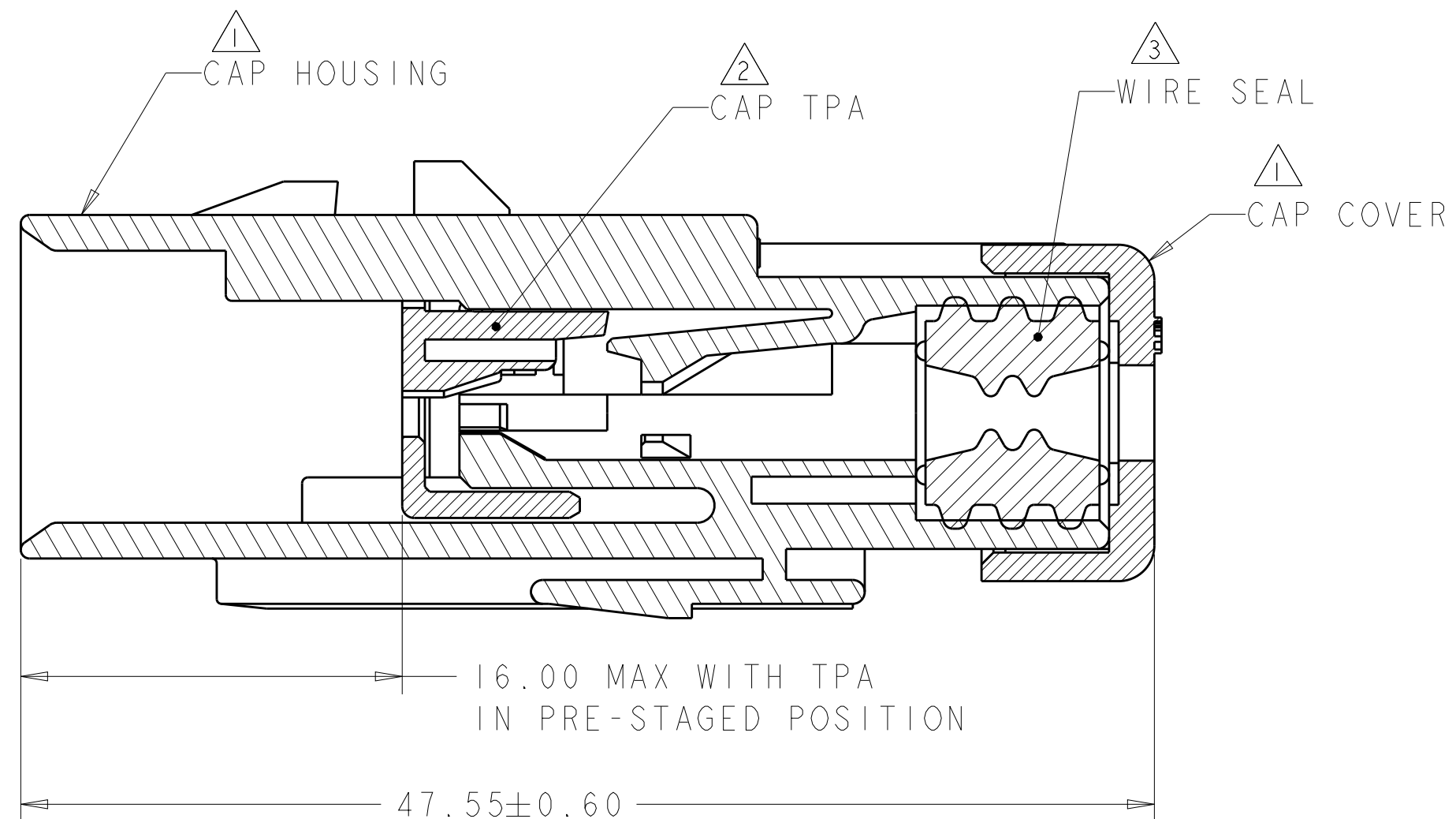
SECTION A-A
