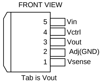
TO263-5L
