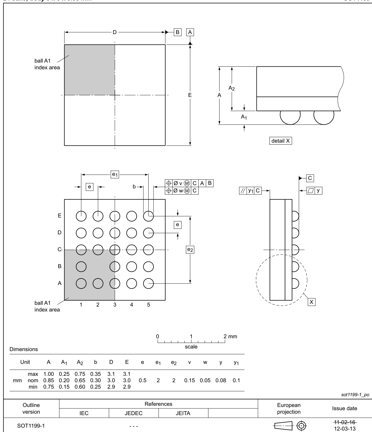
Fig 40. Package outline SOT1199-1 (VFPGA24)
