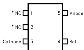
SOT23-5
