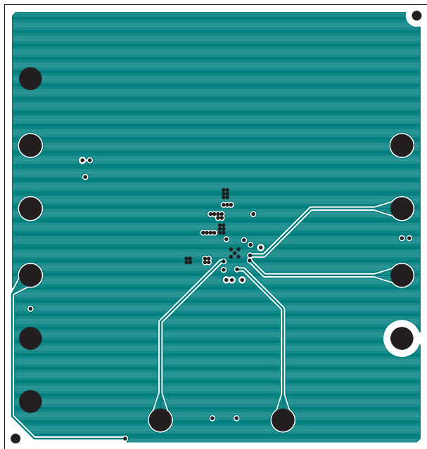
Inner Layer 3
