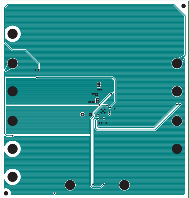
Inner Layer 2
