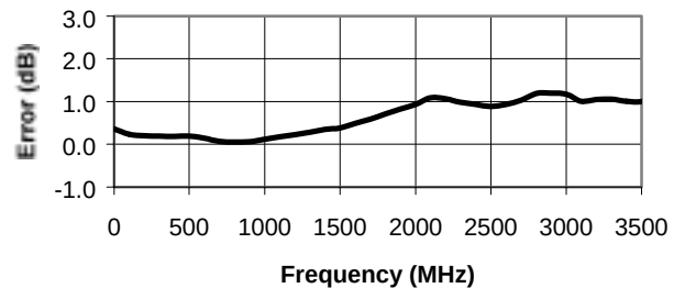
Attenuation Error Maximum Attenuation
