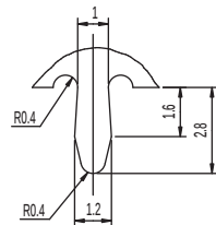
K DETAIL 2:1
