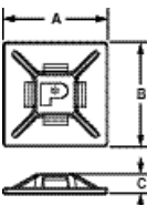
ABMM-A ABMM-AT
