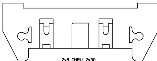
2x8 THRU 2x30 (2x10 SHOWN) STYLE D
