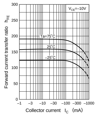
h_{FE} - I_C
