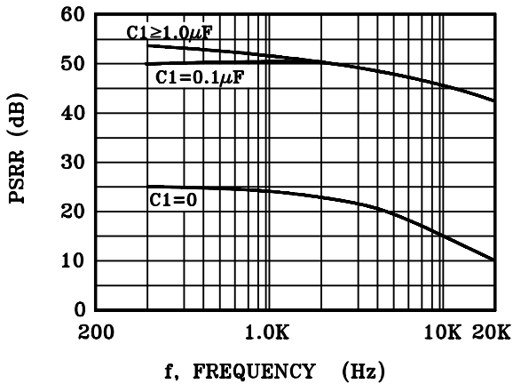
FIGURE4- C_2=10\mu F
