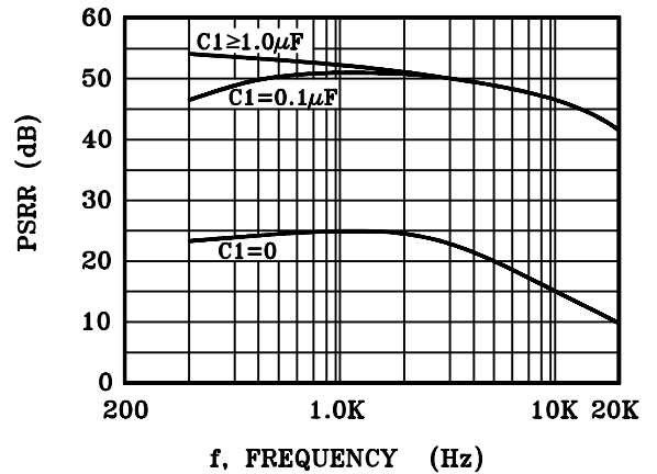
FIGURE5- C_2=5.0\mu F
