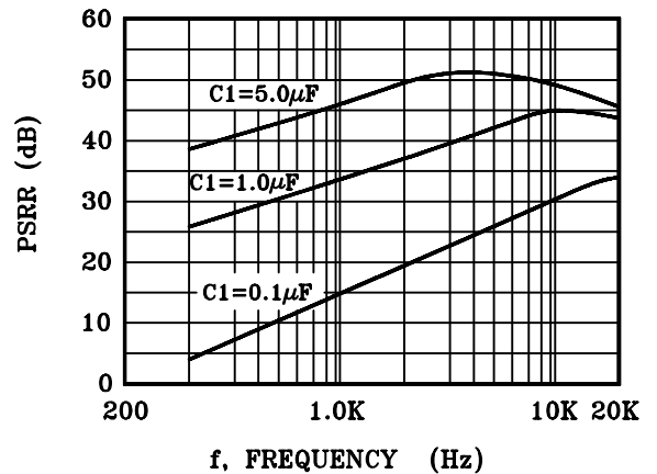
FIGURE7- C_2=0
