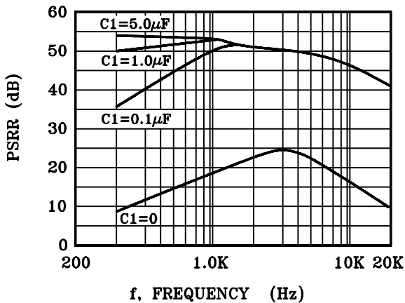
FIGURE6- C_2=1.0\mu F
