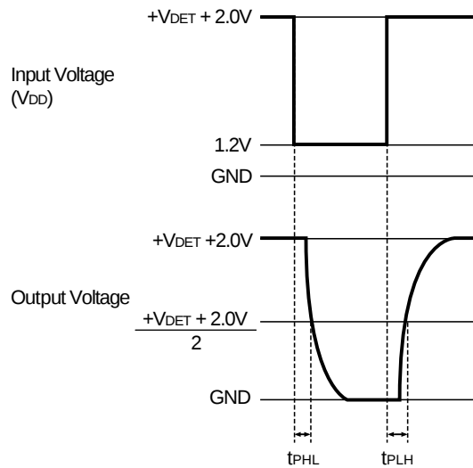
CMOS Output
