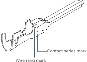
Receptacle Contact
