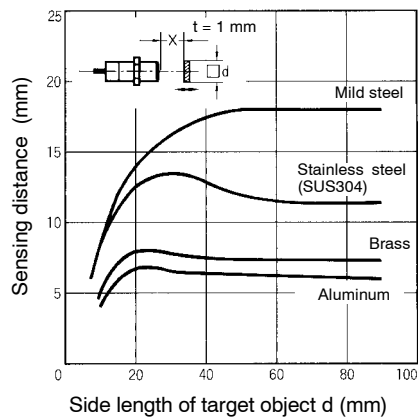
E2E-X18ME□/F□-N E2E-X18MY□-N
