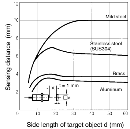
E2E-X10ME□/F□-N
