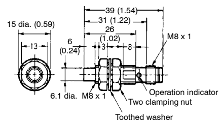
Fig. 21: E2E-X2ME□-M3/F□-M3-N
