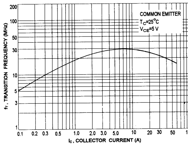
f_T - I_C
