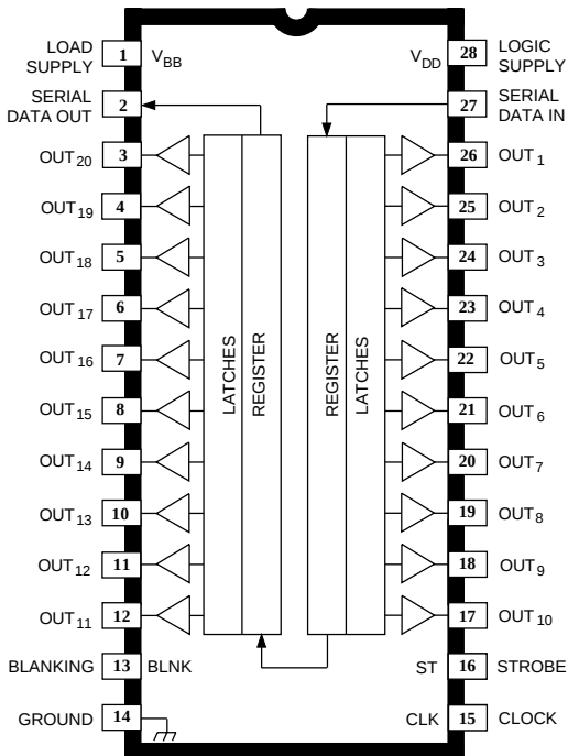
UCN5812AF
