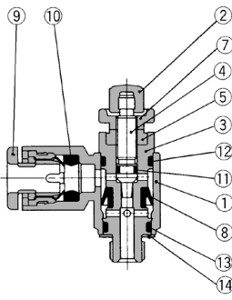
M5 port
