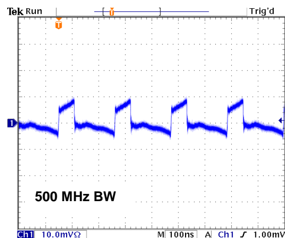
Output Ripple: V_{IN} = 5V , V_{OUT} = 1.2V , I_{out} = 3A
