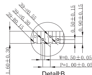
Detail:B Scale:4:1
