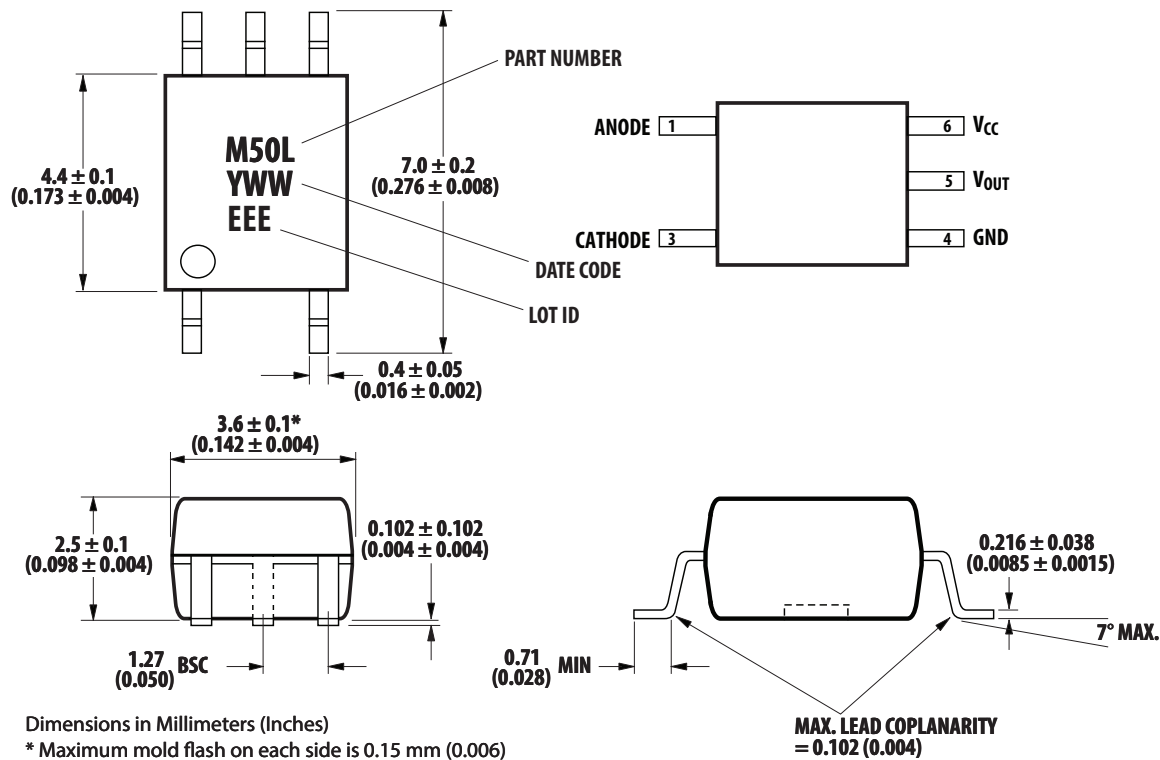
Figure 2 ACPL-M50L SO-5 Package (JEDEC MO-155)
