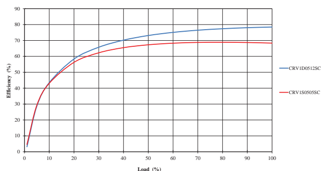
5V Inputs
