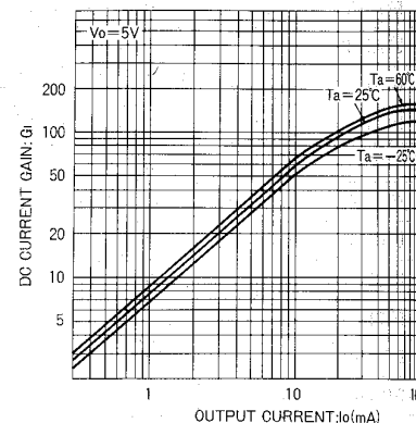
図10 直流電流増幅率 - 出力電流特性
