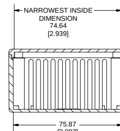
SECTION D-D
