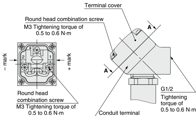
View A-A
