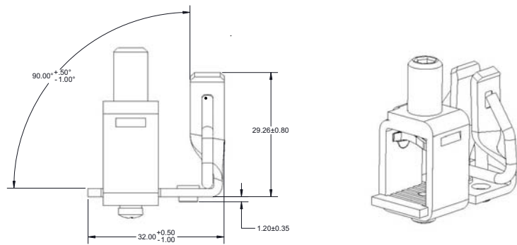
Box lug
