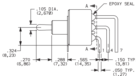
Actuator Shown In Pos. 1
