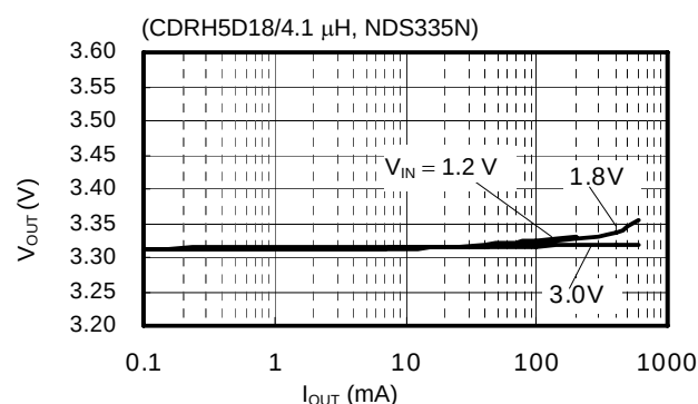
(7) S-8341A33AFT
