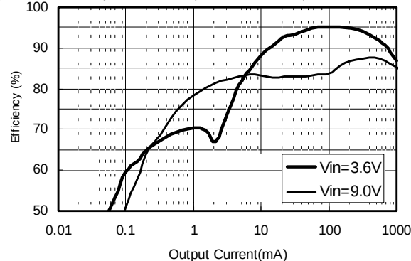
(4) S-8521D30MC
