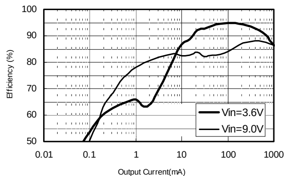
(5) S-8521D30MC
