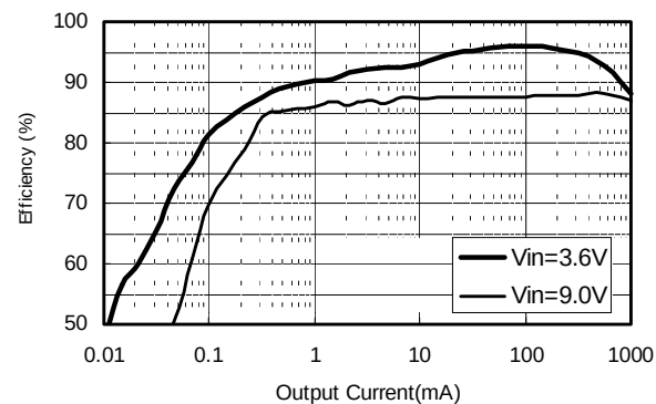
(7) S-8521B50MC
