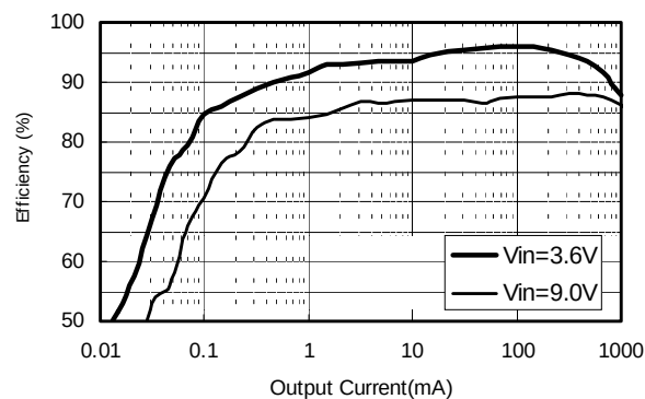
(6) S-8520B50MC
