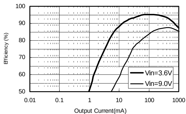
(3) S-8521B30MC
