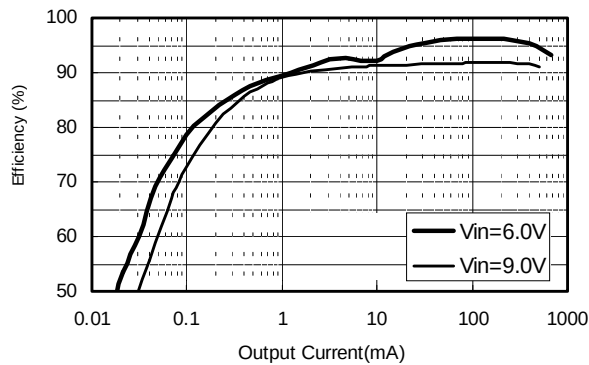
(8) S-8521D50MC
