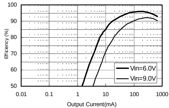
(8) S-8521D50MC
