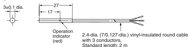
Fig. 1: E2E-CR6□□
