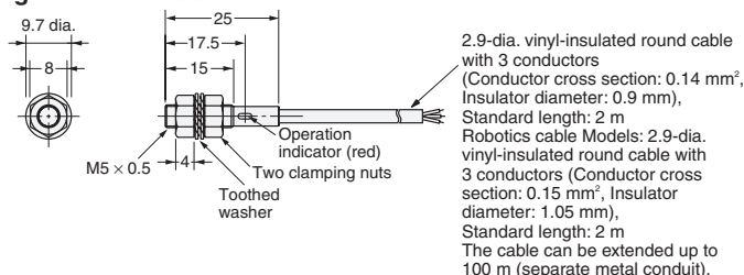
Fig. 4: E2E-X1□□
