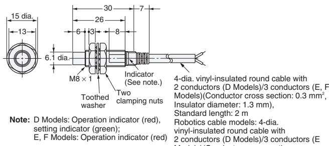
Fig. 6: E2E-X4MD□ E2E-X2ME□/F□
