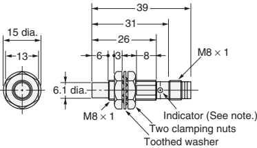
Fig. 29: E2E-X4MD□-M3G/E2E-X2ME□-M3/F□-M3
