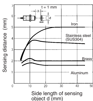
E2E2-X5MC/B E2E2-X5MY
