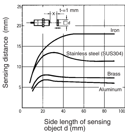
E2E2-X18MC/B E2E2-X18MY
