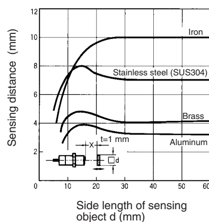
E2E2-X10C/B E2E2-X10Y
