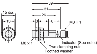
Fig. 28: E2E-X2D□-M3G/E2E-X1R5E□-M3/F□-M3
