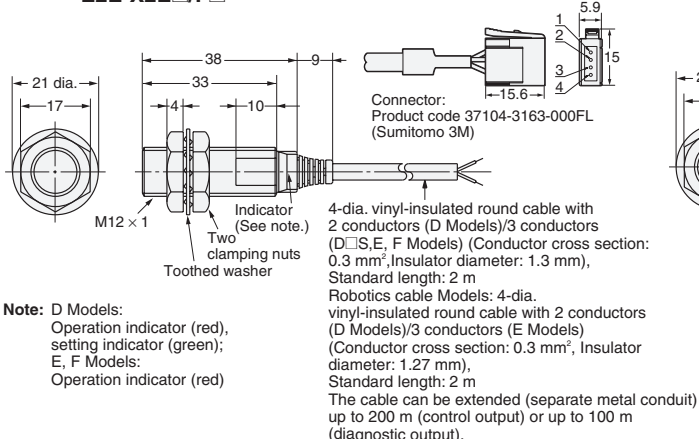
Fig. 9: E2E-X3D□-N E2E-X2E□/F□
