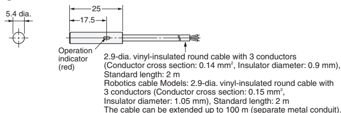
Fig. 4: E2E-X1□□
