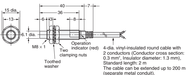
Fig. 10: E2E-X8MD□ E2E-X5ME□/F□
