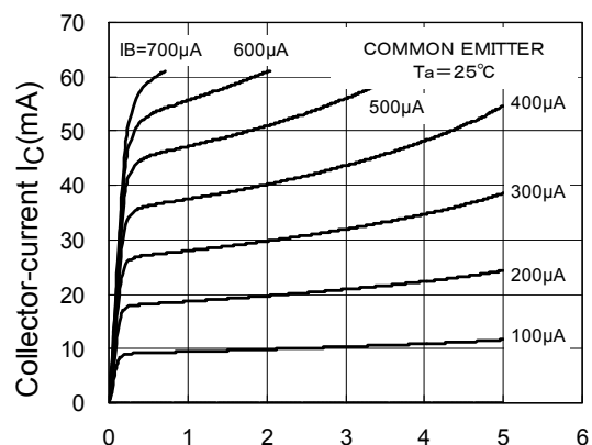
I_C-V_{CE}
