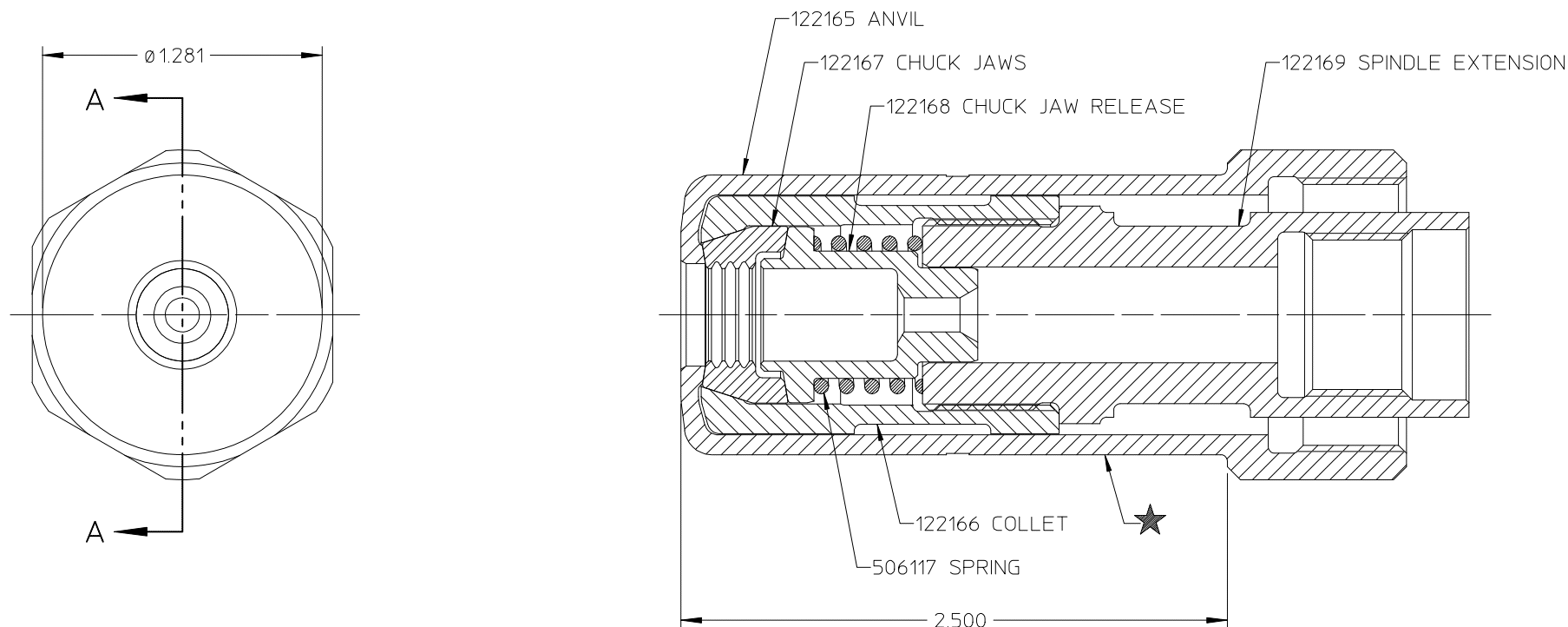
SECTION A-A
