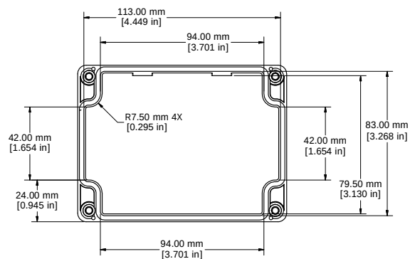
LID - INSIDE
