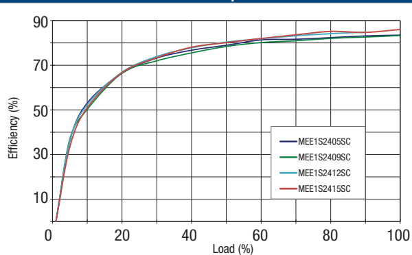
24V Input
