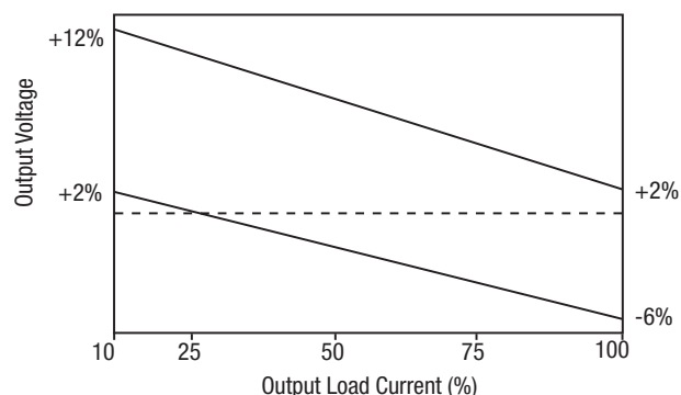
9V Output
