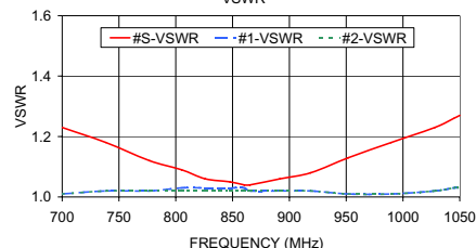
ZN2PD-920W VSWR
