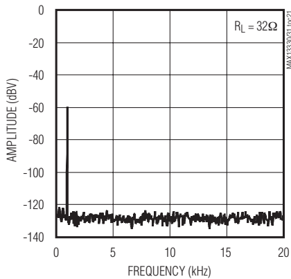
OUTPUT FFT
