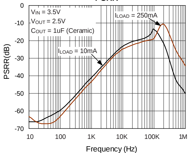
PSRR
