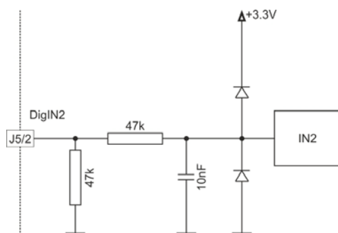
Abbildung 3-11 DigIN2 Schaltung
