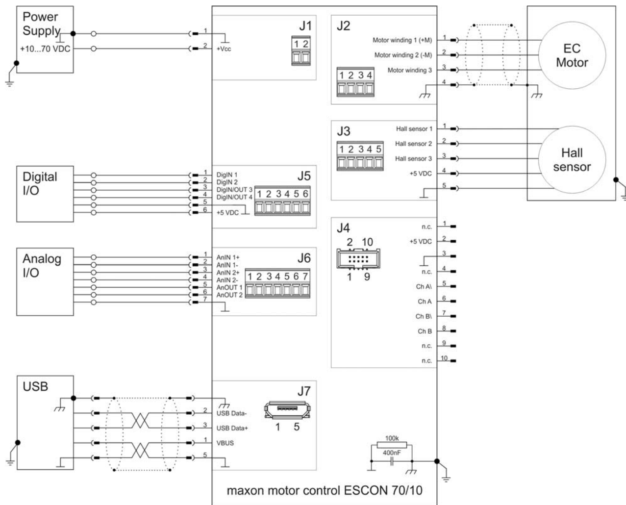
Abbildung 4-25 maxon EC motor mit Hall-Sensoren (J2 / J3)
