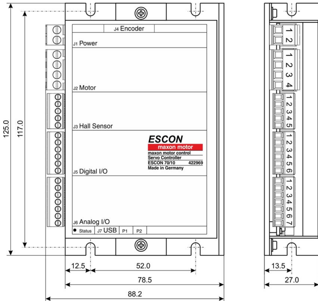
Abbildung 2-1 Massbild [mm]
