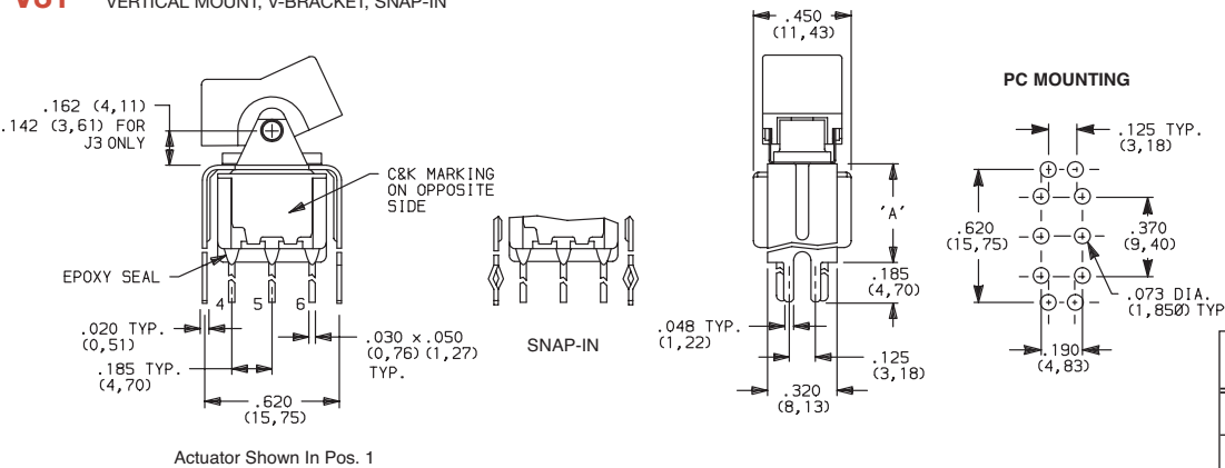
7201J1_BE2 DPDT
