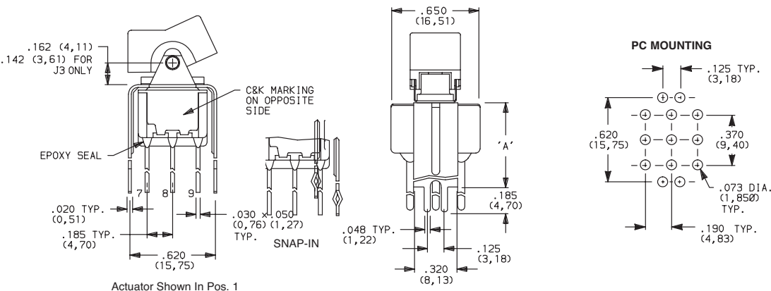
7301J1_BE2 3PDT
