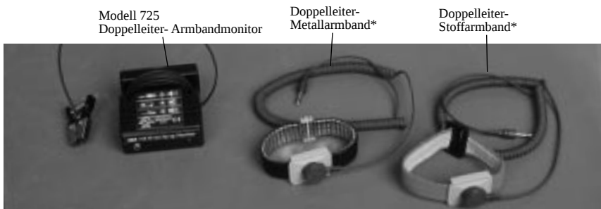
Abbildung 1 - 3M Modell 725 Armbandmonitor mit Doppelleiter-Armbändern
