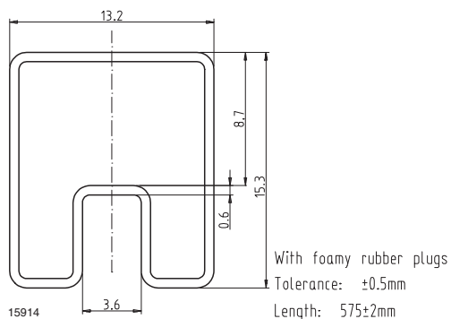
Fig. 16 - CNY65Exi
