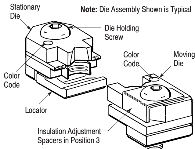
CRIMPING DIE ASSEMBLIES
