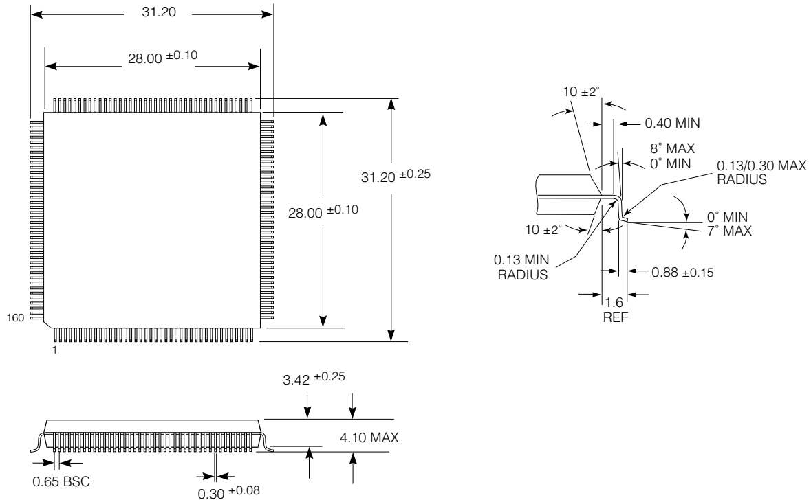
Fig. 14 160 Pin MQFP
