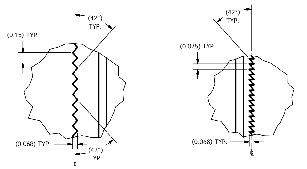
DETAIL G APERTURE RIGHT EDGE SCALE 60 : 1
