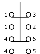
DPDT Non ILL SCHEMATIC
