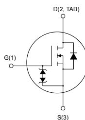
DPAK
