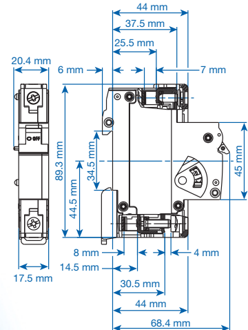
Dimensions UA120L
