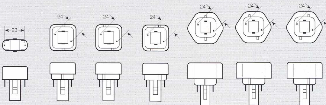
G23 Sheet 7004-69
