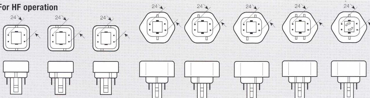
G24q-1 Sheet 7004-78
