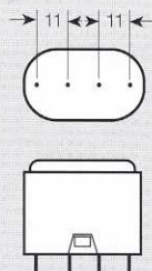
2G11 Sheet 7004-82
