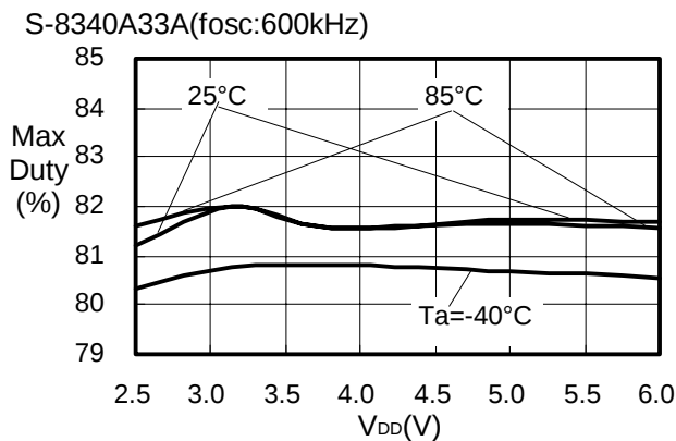
(14) MaxDuty—V DD
