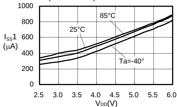
(3) I_{SSS} — V_{DD}
