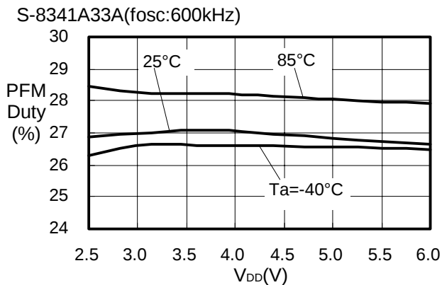
(15) PFMDuty—V DD
